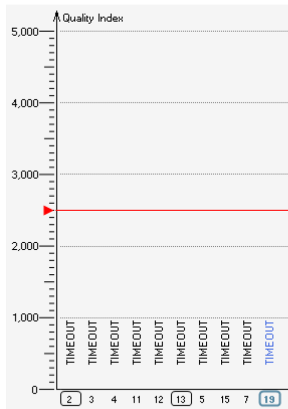
Messung am Busende (Adr. 19)
