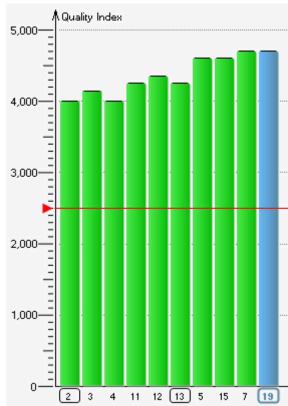
Messung am Busende (Adr. 19) bei 1.5 Mbit/s
