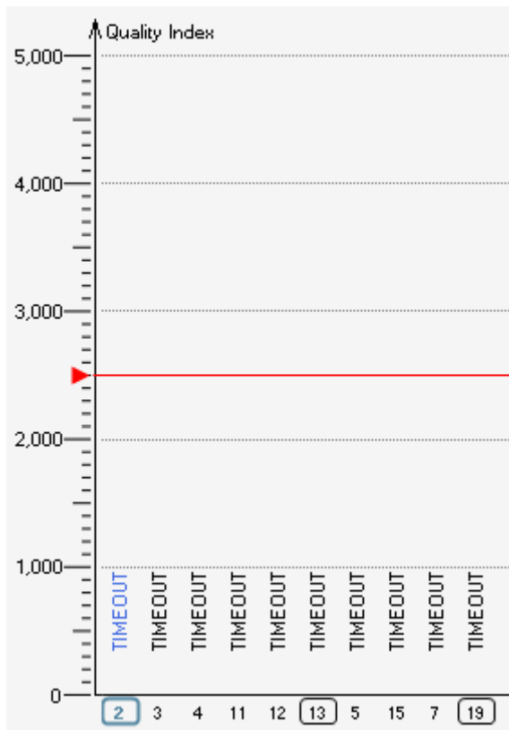
Messung am Busanfang (Adr. 2)
