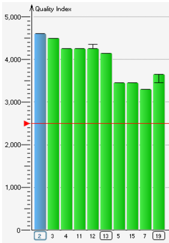
Messung am Busanfang (Adr. 2) bei 1.5 Mbit/s
