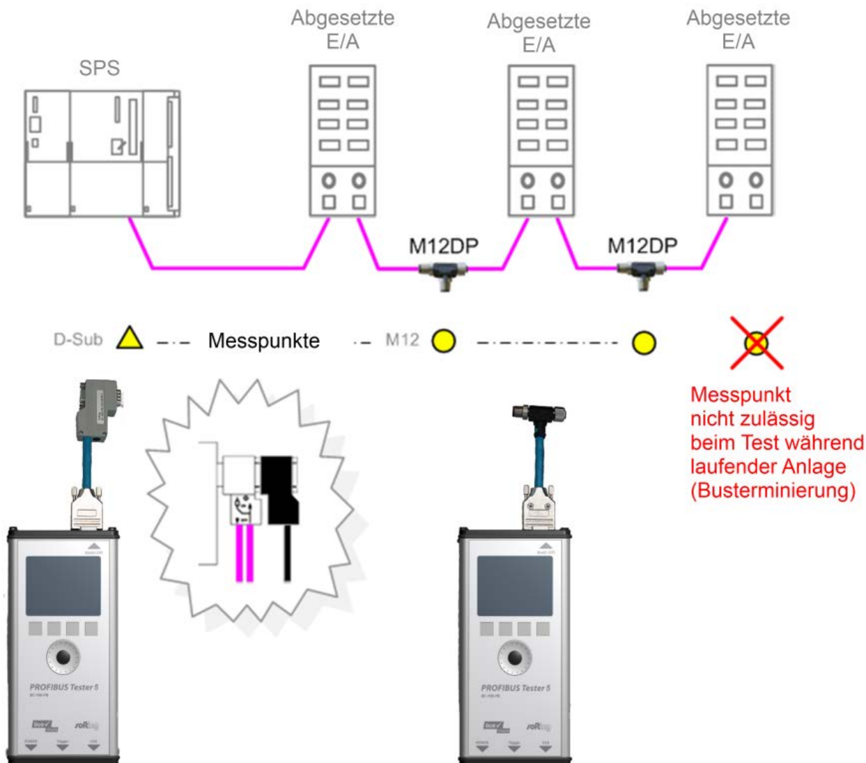
Abbildung 19: Messpunkt in laufenden Anlagen mit Anschlussart M12
