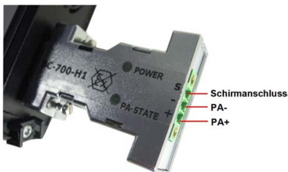
Abbildung 23: PROFIBUS-PA Pinbelegung
