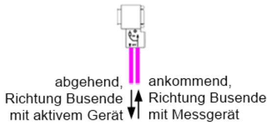
Abbildung 21: Kontrolle der Anschlussrichtung am D-Sub-Stecker - nur Topologiemessung
