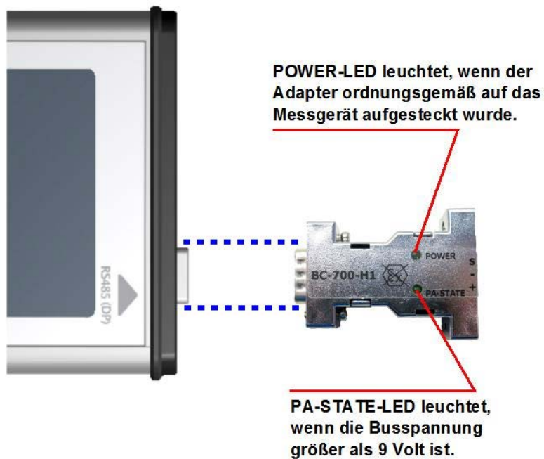
Abbildung 22: Anschluss des PA-Adapters an das Testgerät
