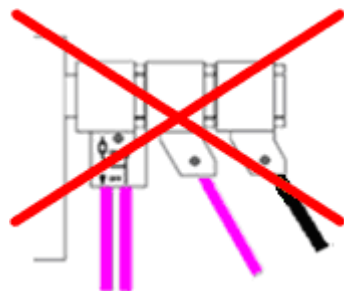
Abbildung 14: Unzulässige Kaskadierung von D-Sub-Steckern
