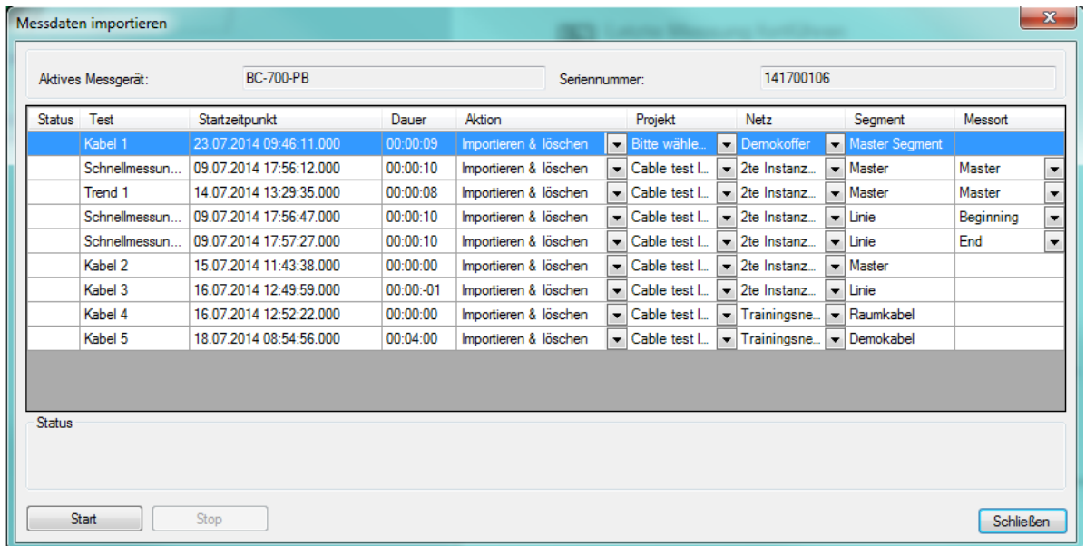
Abbildung 29: Messdaten importieren
