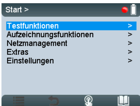
Abbildung 25: Startbildschirm
