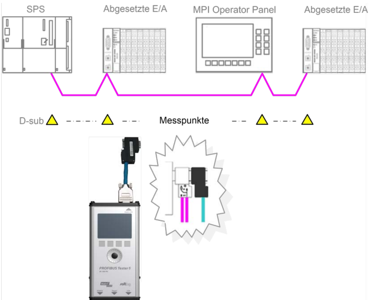
Abbildung 17: Messpunkte für das D-Sub-Adapterkabel
